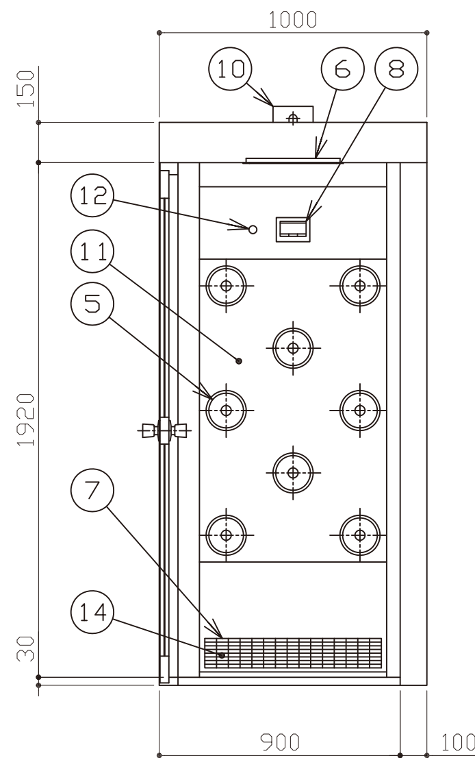
A-A断面
